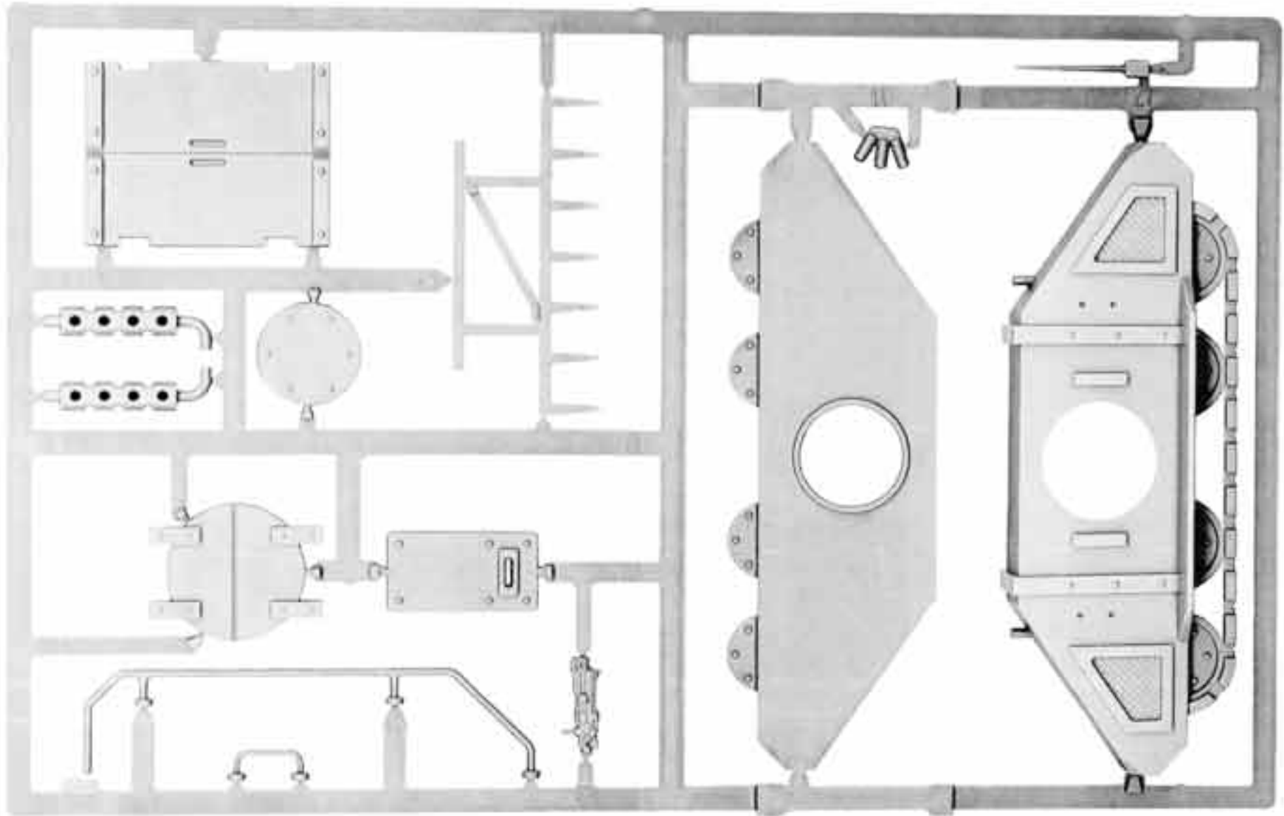
RHINO TRACK SPRUE 99399999054 SHOWN AT 70% ACTUAL SIZE
